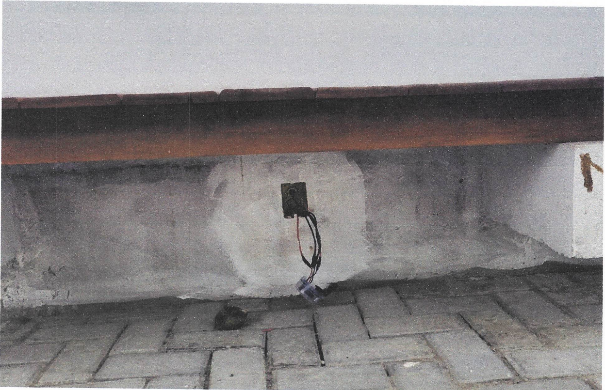
FOTO 12 - CABO DE COBRE FLEXÍVEL ISOLADO, 1,5 MM 2 , ANTI-CHAMA 450/750 V, PARA CIRCUITOS TERMINAIS - FORNECIMENTO E INSTALAÇÃO. AF_12/2015.
